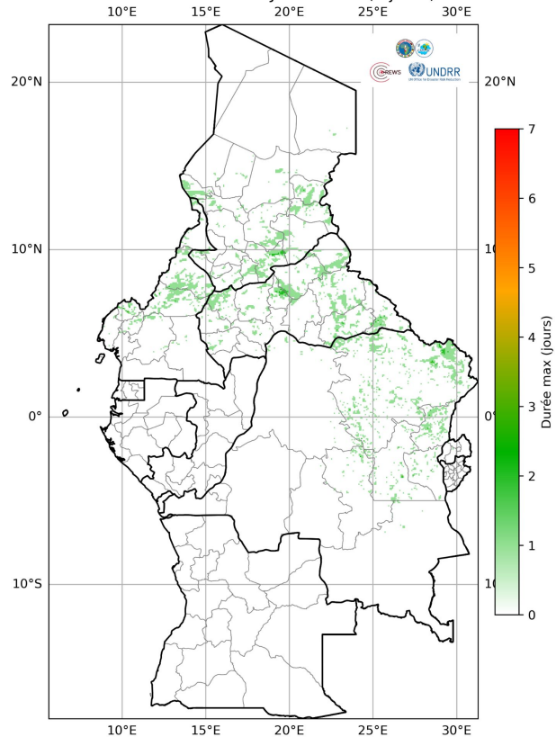
Wet Spells WRF ( \geq 50 mm/jour) Semaine du 13 au 19 Juillet 2026 (7 jours)
