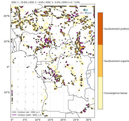
ITVC - Indice de Temps Violent Convectif Échéance : 2026-07-15 00:00 UTC
