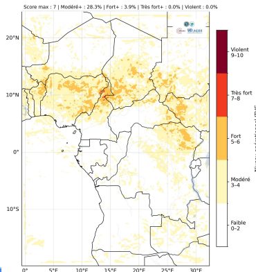
ITVC - Indice de Temps Violent Convectif Échéance : 2026-07-15 00:00 UTC
