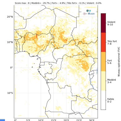
ITVC - Indice de Temps Violent Convectif Échéance : 2026-07-16 00:00 UTC
