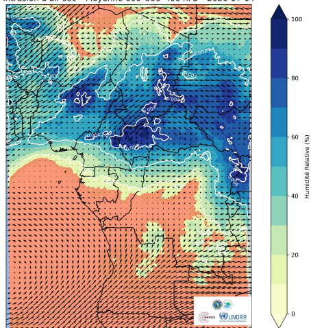
Intrusion d'air sec - Moyenne 600-500-400 hPa - 2026-07-14
