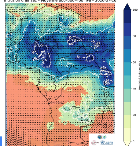
Intrusion d'air sec - Moyenne 600-500-400 hPa - 2026-07-16
