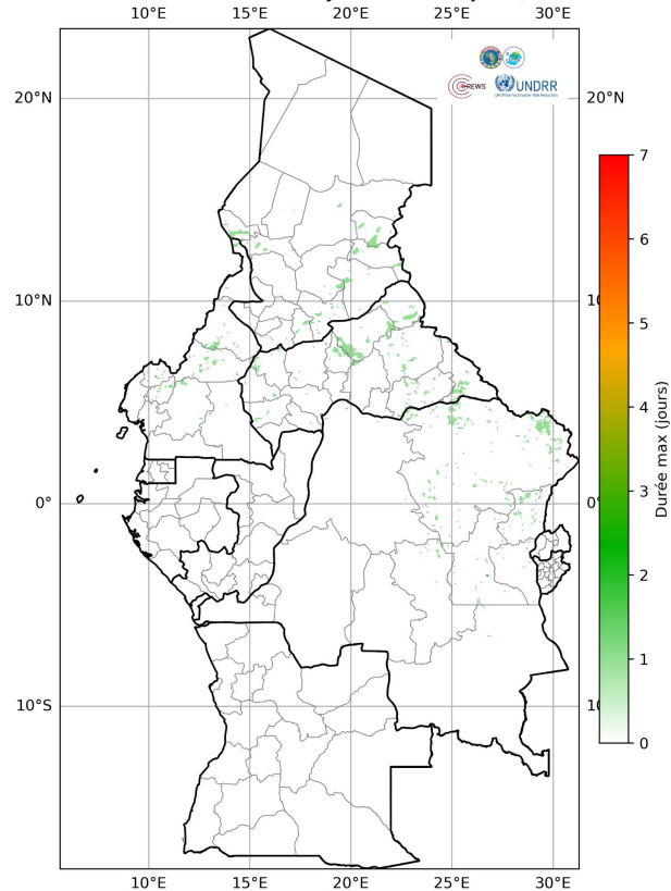
Wet Spells WRF ( \geq 75 mm/jour) Semaine du 13 au 19 Juillet 2026 (7 jours)
