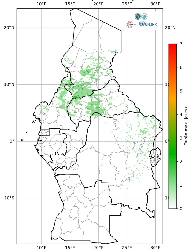
Wet Spells WRF ( \geq 50 mm/jour) Semaine du 20 au 26 Juillet 2026 (7 jours)
