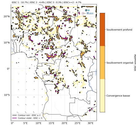
ITVC - Indice de Temps Violent Convectif Échéance : 2026-07-14 00:00 UTC
