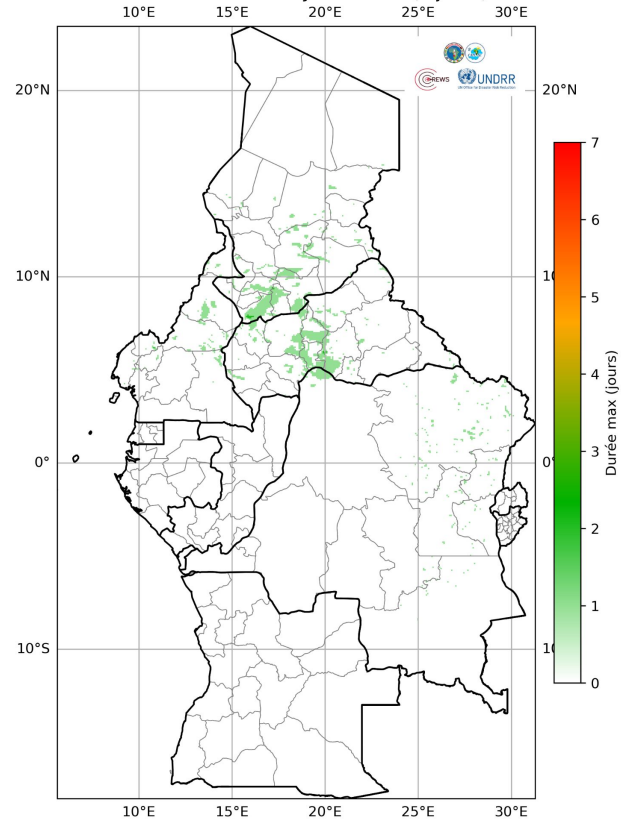
Wet Spells WRF ( \geq 75 mm/jour) Semaine du 20 au 26 Juillet 2026 (7 jours)
