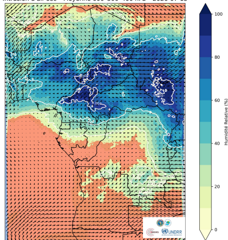
Intrusion d'air sec - Moyenne 600-500-400 hPa - 2026-07-15
