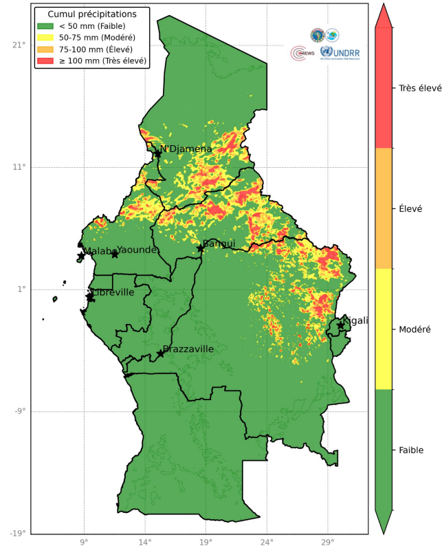
Carte de vigilance du 2026-07-13 au 2026-07-19
