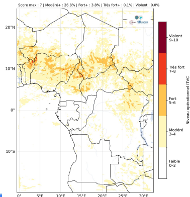
ITVC - Indice de Temps Violent Convectif Échéance : 2026-07-14 00:00 UTC
