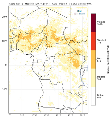
ITVC - Indice de Temps Violent Convectif Échéance : 2026-07-16 00:00 UTC
