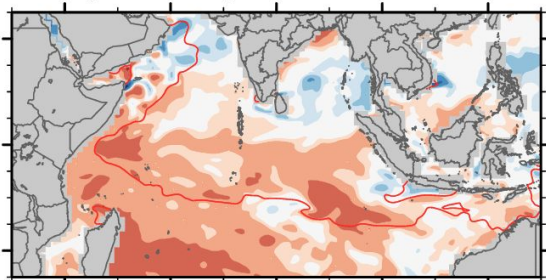
16-Aug to 22-Aug
