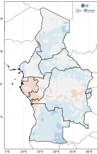
Anomalie d'humidité du sol Semaine du 17-23 août 2026
