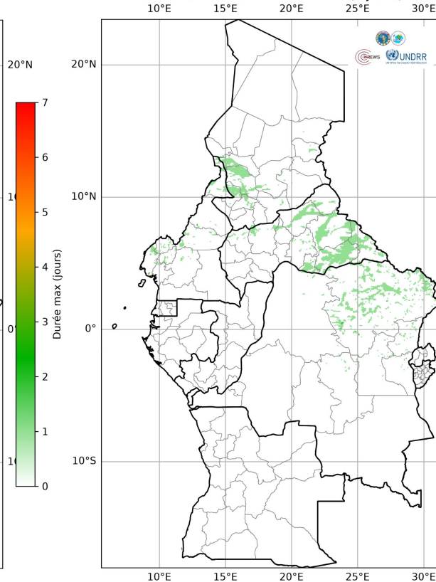
Wet Spells WRF ( \geq 75 mm/jour) Semaine du 17 au 23 Août 2026 (7 jours)
