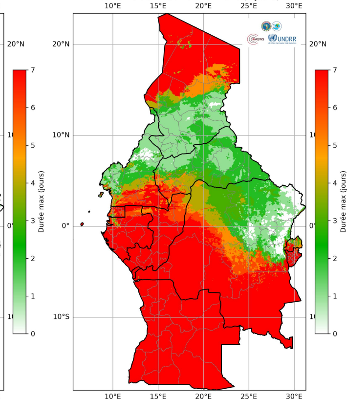
Dry Spells WRF ( < 1 mm/jour) Semaine du 17 au 23 Août 2026 (7 jours)
