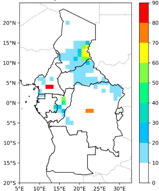
R99p : Du 01-10 août
