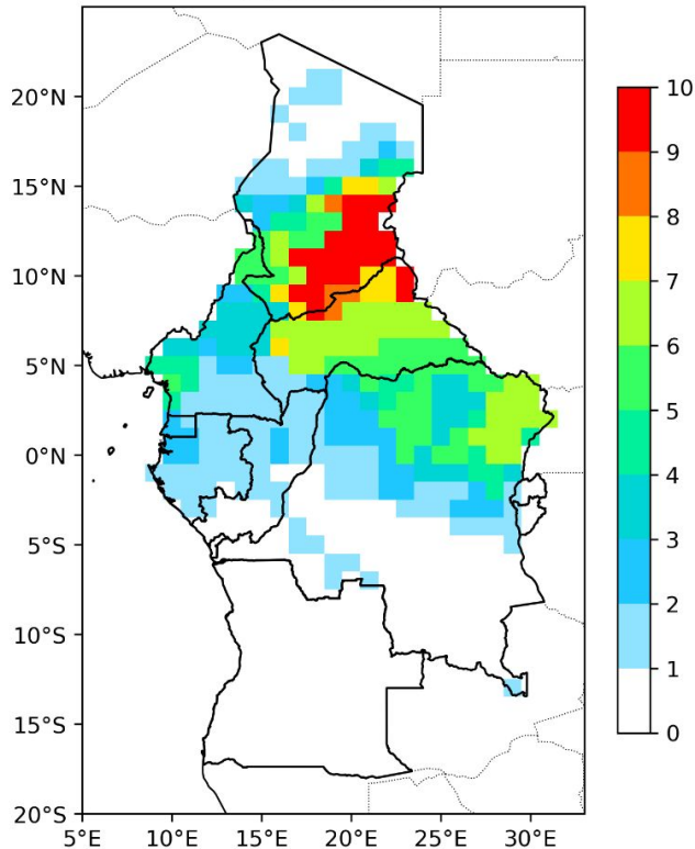
Nombres de Jours Humides Consécutifs Du 01-10 août
