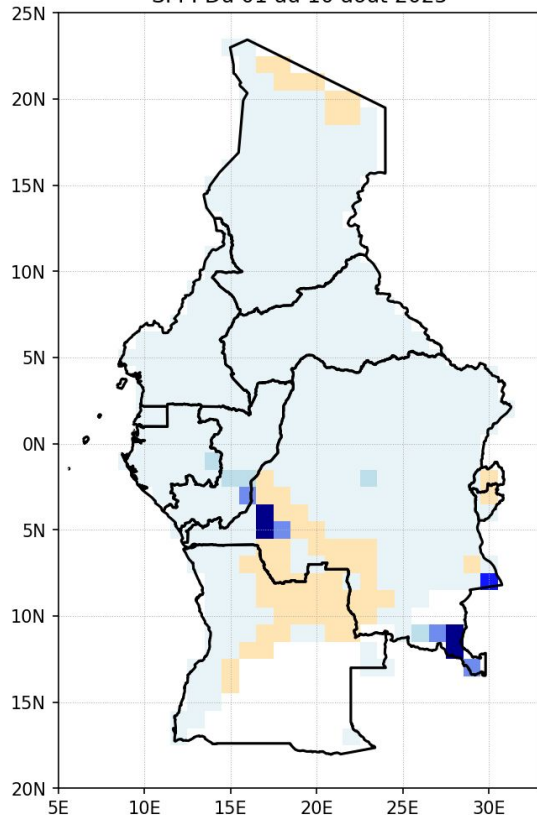
SPI : Du 01 au 10 août 2025
