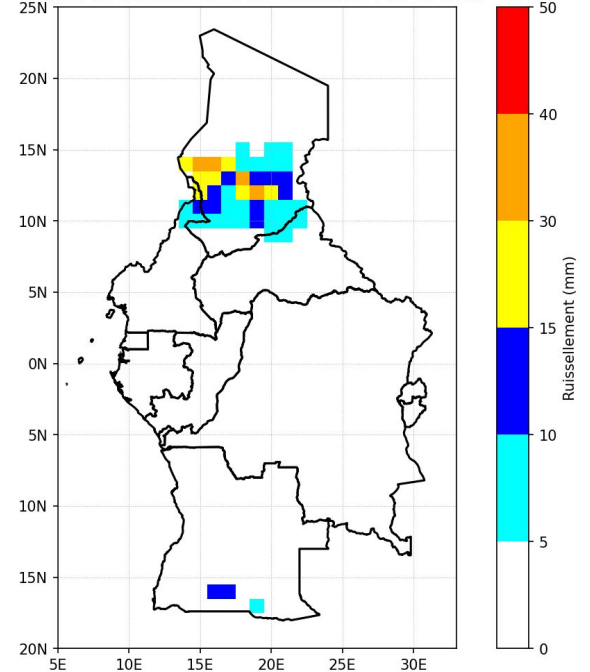
Indice de Ruissellement de subsurface : 21-30 aout
