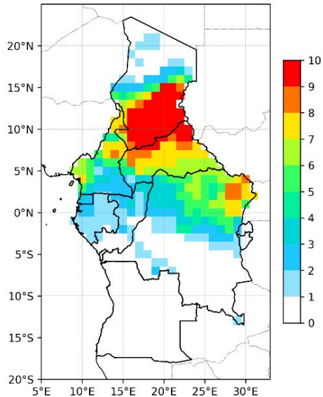
Indice des Jours Humides ( \geq 1 mm) 01-10 août
