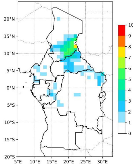
Indice des Jours Humides ( \geq 10 mm) 01-10 août
