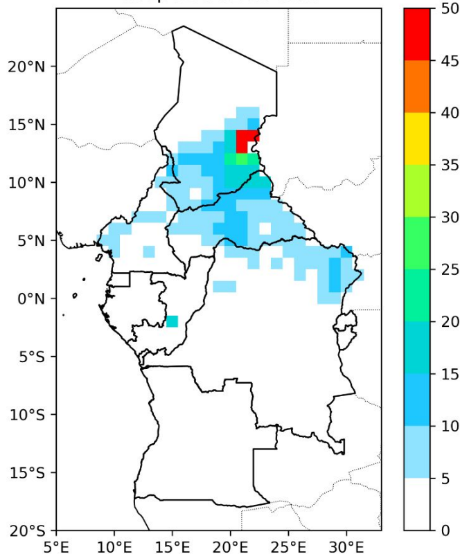
R90p : Du 01-10 août
