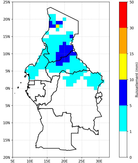
Indice de Ruissellement de surface : 11-20 aout
