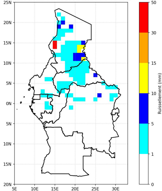
Indice de Ruissellement de surface : 01-10 aout
