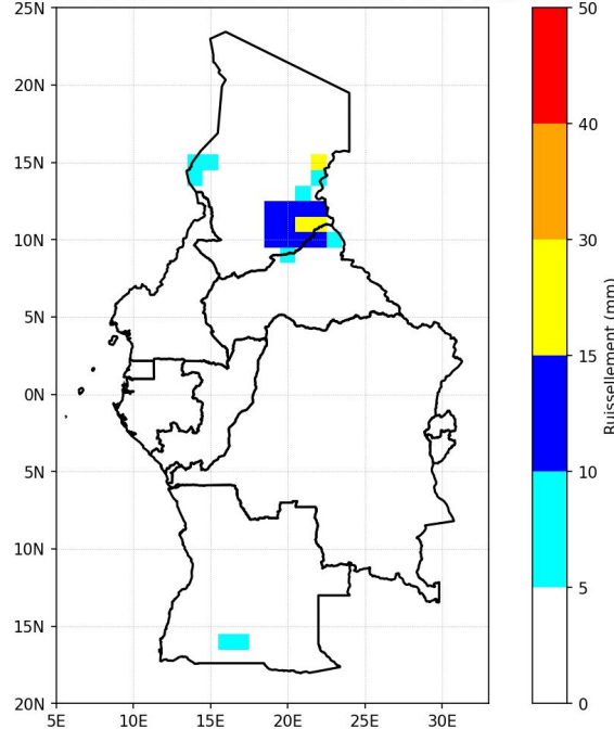
Indice de Ruissellement de subsurface : 11-20 aout
