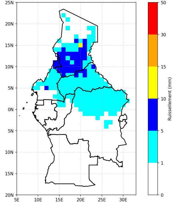
Indice de Ruissellement de surface : 21-30 aout
