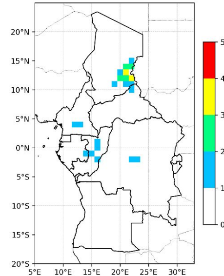
Indice des Jours Humides ( \geq 20 mm) 01-10 août
