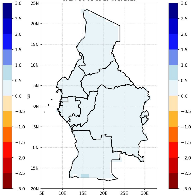
SPEI : Du 01 au 10 août 2025
