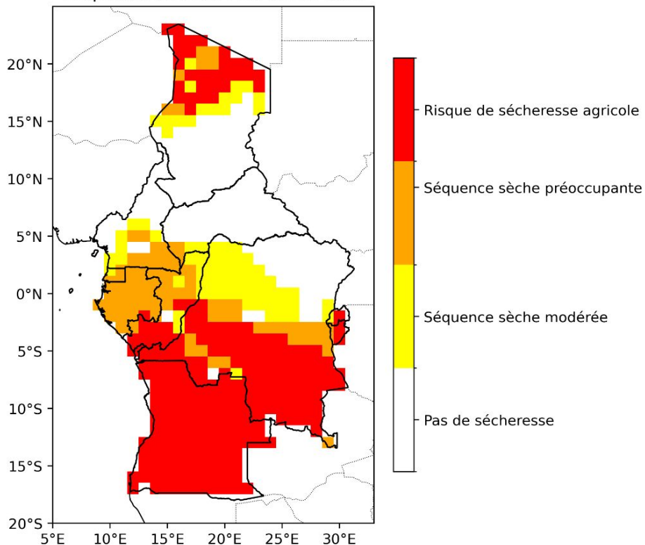
Séquences sèches : Du 01-10 août
